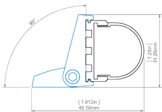
GIZA profile with G-L cover and REGIP-UV mounting bracket profil GIZA z oslóną G-L oraz mocowníkem REGIP-UV
