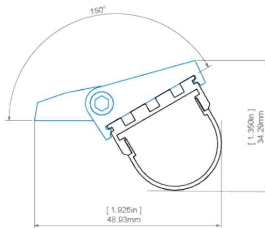
GIZA profile with G-L cover and REGIP-UV mounting bracket profil GIZA z oslóną G-L oraz mocowníkem REGIP-UV
